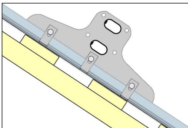
Монтаж на Сمارт Фальц ПРО, высота замка 32 мм
