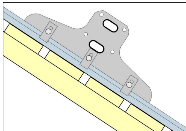
Монтаж на двойной стоячий фальц, высота замка 25 мм
