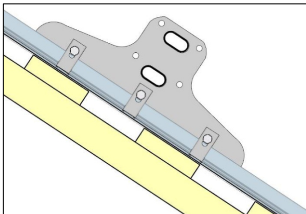
Монтаж на Смарт Фальц ПРО, высота замка 32 мм
